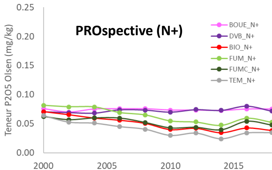
Teneur du sol en P_2O_5 Olsen
